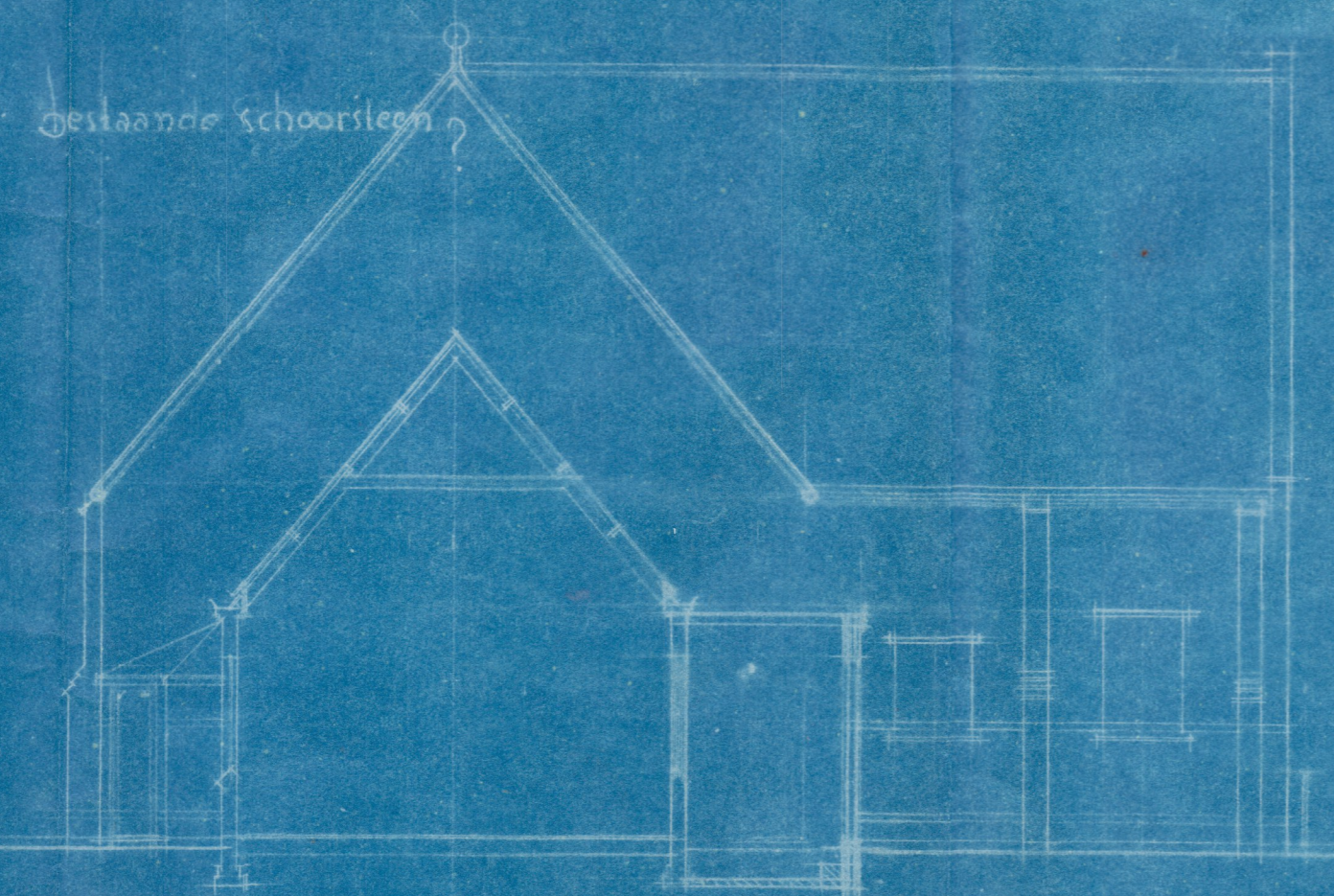
DOORSNEDEN A.A
