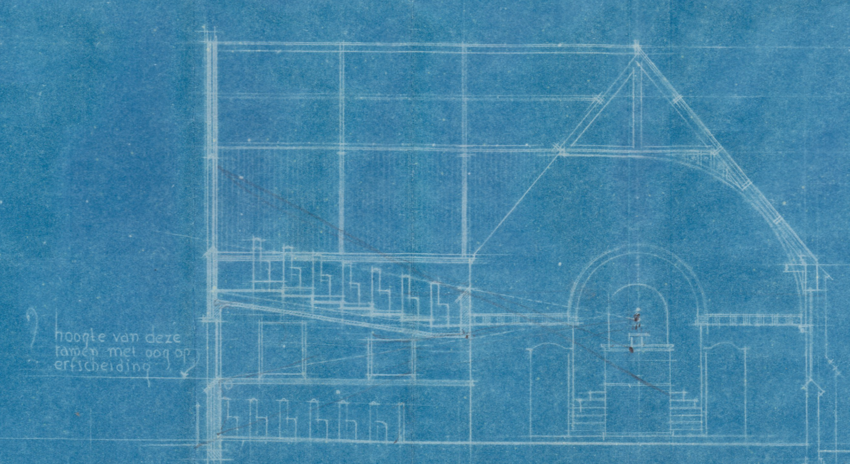
DOORSNEDEN C.C.
