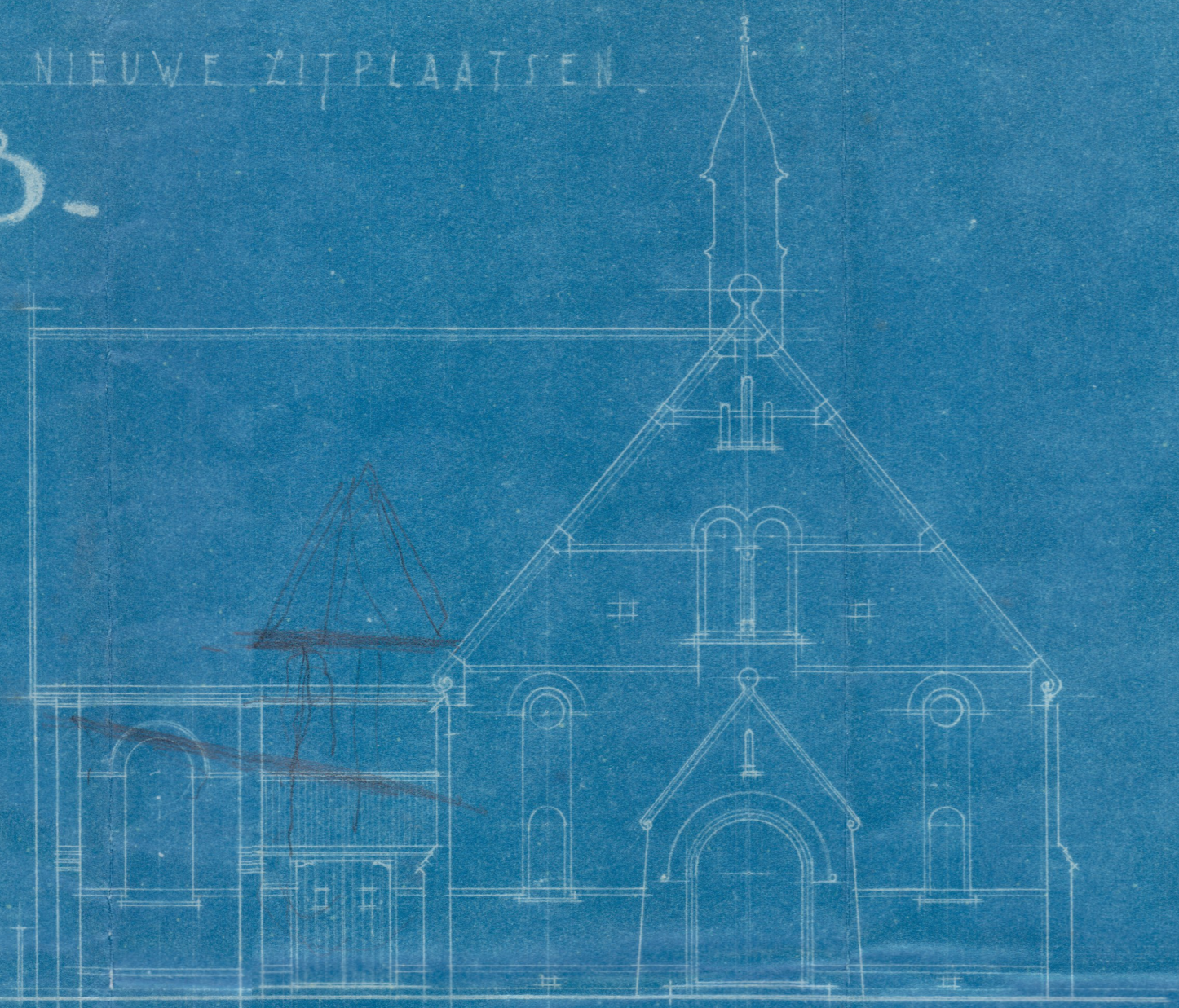
VOORGEVEL
